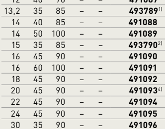
Élszintbemaró golyócsapággal HW s = 8
